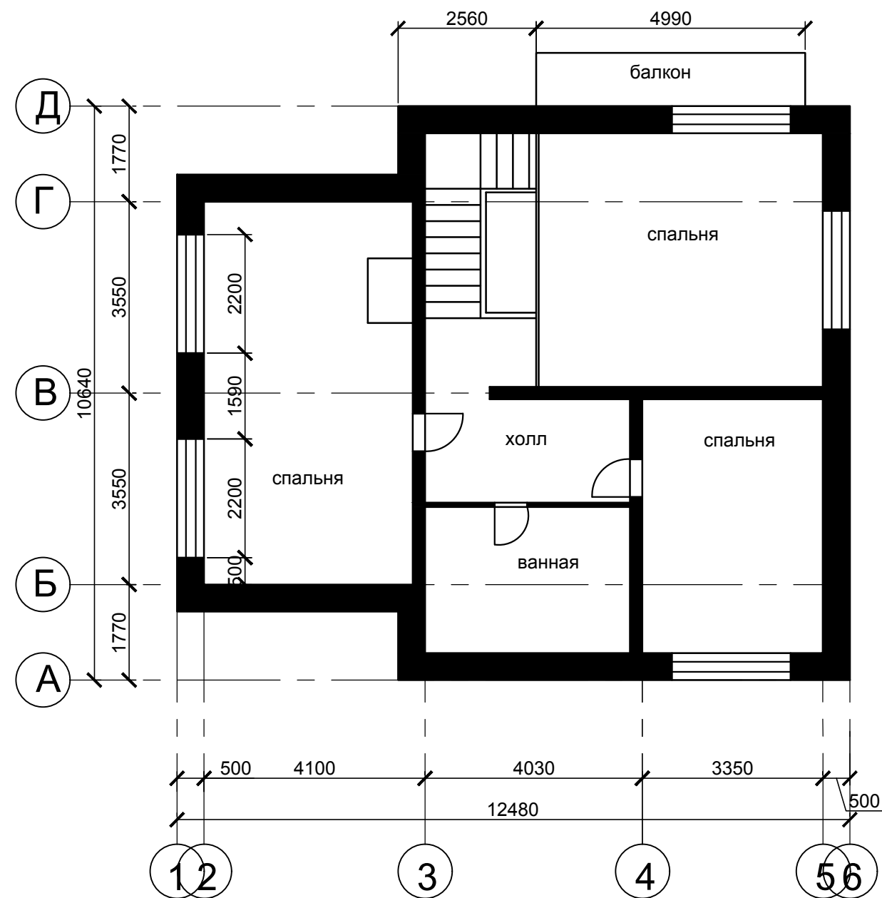
План на отм. 3.000 мансарда
